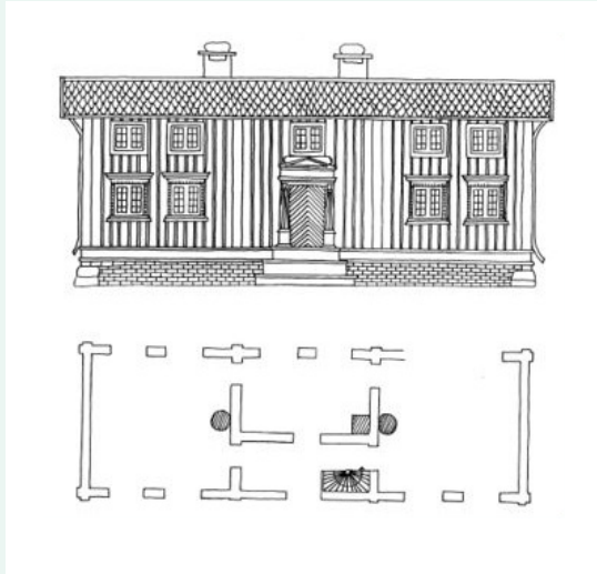
Skisse av midtkammersbygning .
